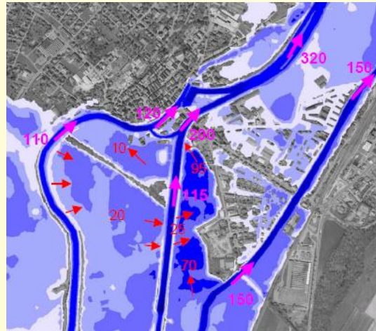
Zustand vor Bau (überschwemmte Flächen bei HQ100)
